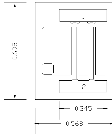
正视图
