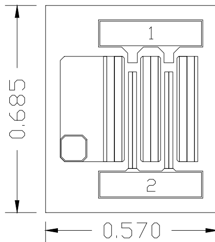
正视图
