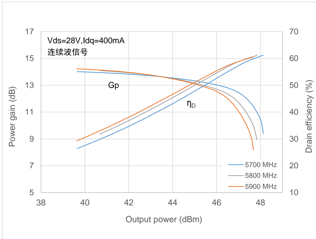
增益, 漏极效率 vs.输出功率 (连续波)
